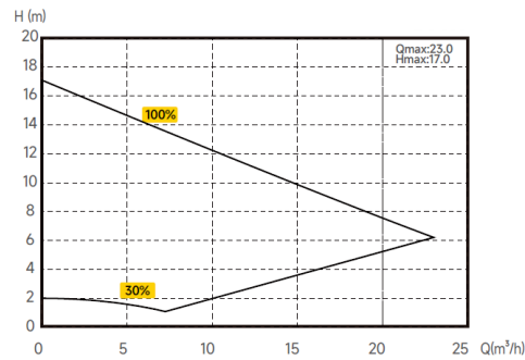
prestatiecurve
